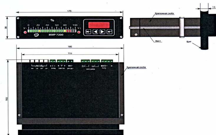
Рисунок 1.в - Внешний вид МИР-7200 исполнение 02
