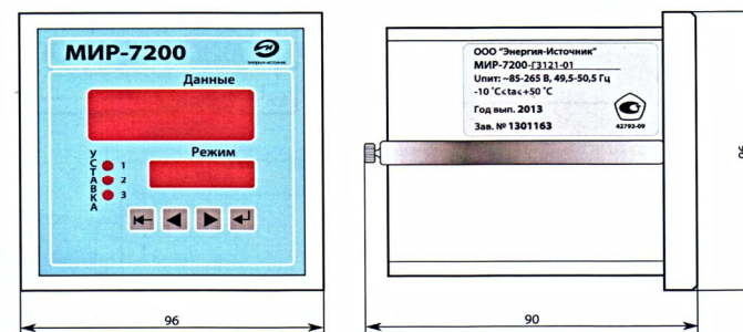
Рисунок 1.б - Внешний вид МИР-7200 исполнение 01
