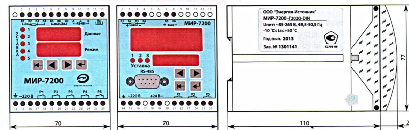
Рисунок 1.а - Внешний вид МИР-7200 исполнение DIN
