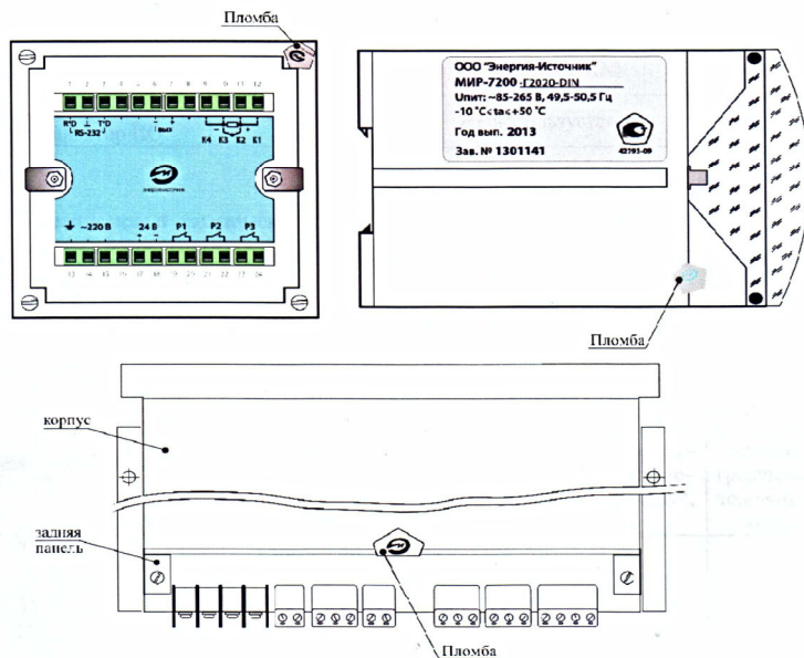
Рисунок 2 - Схема пломбировки МИР-7200
